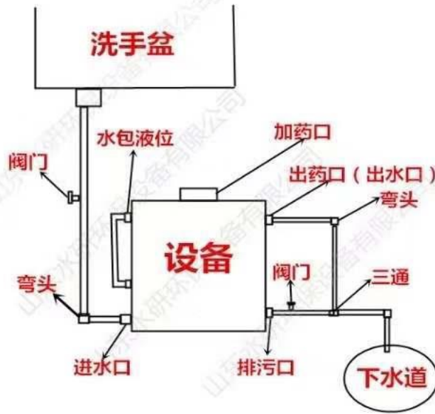
图 4-1 缓释消毒器设备图
